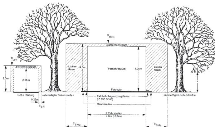
S s = seitlicher Sicherheitsraum S o = oberer Sicherheitsraum R = Radfahrer Kfz = Kraftfahrzeug * Kronenansatz in Abhängigkeit von Baumart, Wuchsform des Baumes, angrenzende Nutzung und Topographie (z. B. bei Einschnitt)
